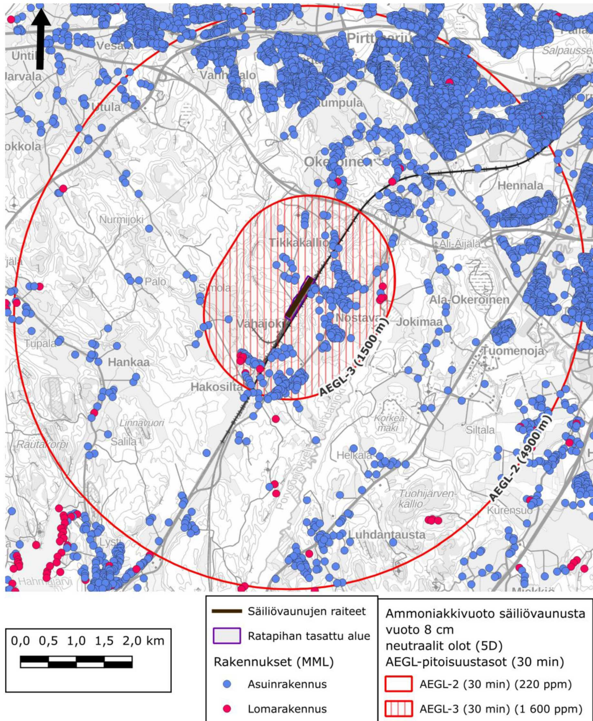
Kuva 38. Ammoniakkivuodon aiheuttamat AEGL-tasojen etäisyydet, kun vedetöntä ammoniakkia vuotaa säiliövaunun pohjalta. Vuodon koko 8 cm, ammoniakkin lämpötila +15 °C. Neutraalit olot (luokka D), tuulen nopeus 5 m/s ja ilman lämpötila +15 °C.
