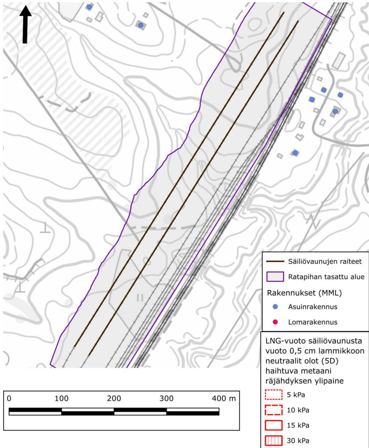
Kuva 28. Vuodon koko 0,5 cm. Neutraalit olot (luokka D), tuulen nopeus 5 m/s ja ilman lämpötila +15 °C. Räjähdystä ei tapahdu, koska kaasupilvessä syttymisraja ei ylitä minuutin vuodon jälkeen.
