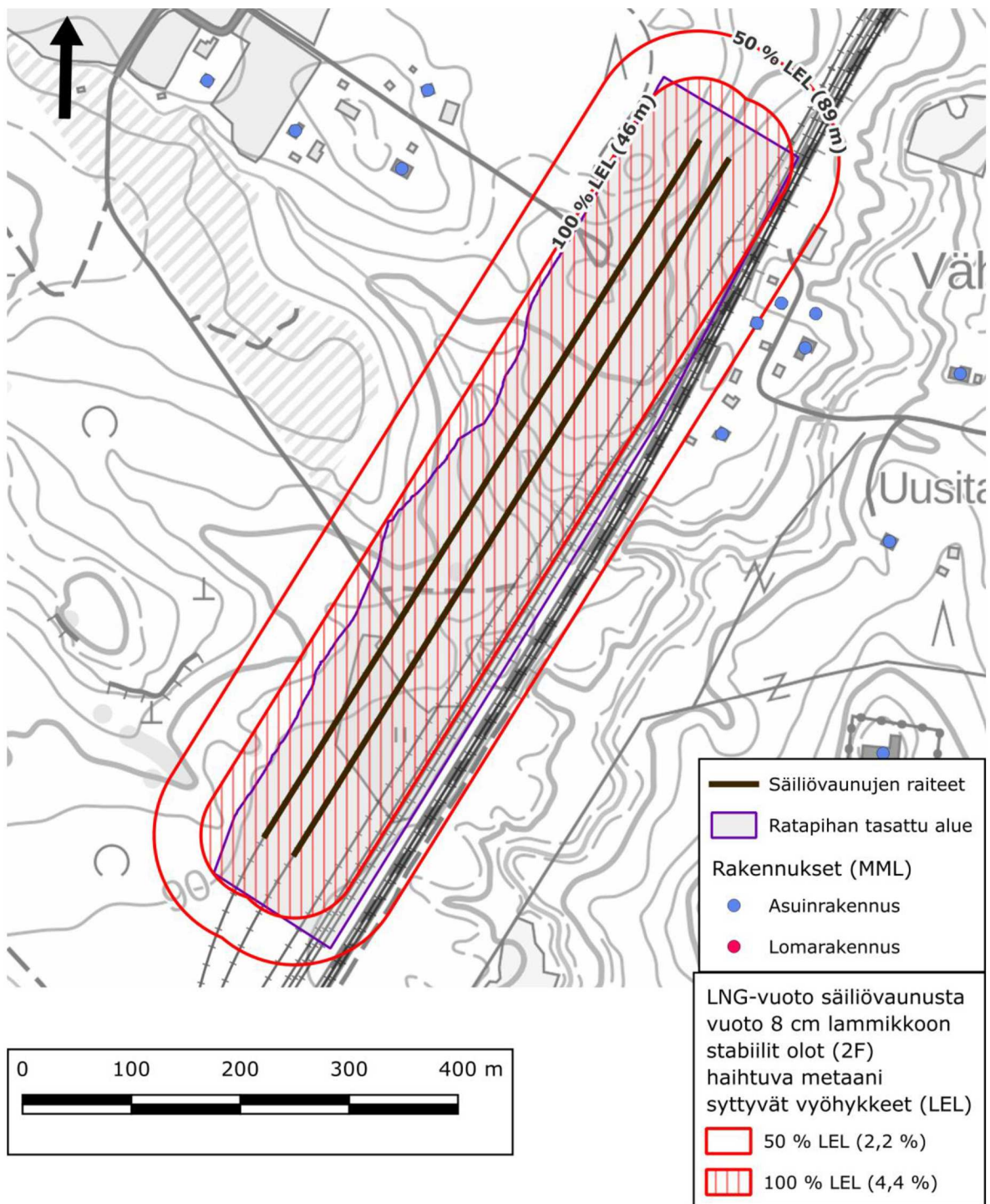
Kuva 21. Syttyvät vyöhykkeet metaanin haihtuessa vuotaneen LNG:n muodostamasta lammikosta. Vuodon koko 8 cm. Stabiilit olot (luokka F), tuulen nopeus 2 m/s ja ilman lämpötila +15 °C.
