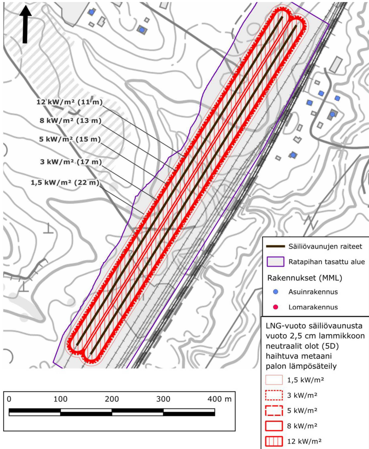
Kuva 24. Lämpösäteilyn tehotasojen vyöhykkeet, kun LNG:n muodostamasta lammikosta haihtuva metaani palaa. Vuodon koko 2,5 cm. Neutraalit olot (luokka D), tuulen nopeus 5 m/s ja ilman lämpötila +15 °C.
