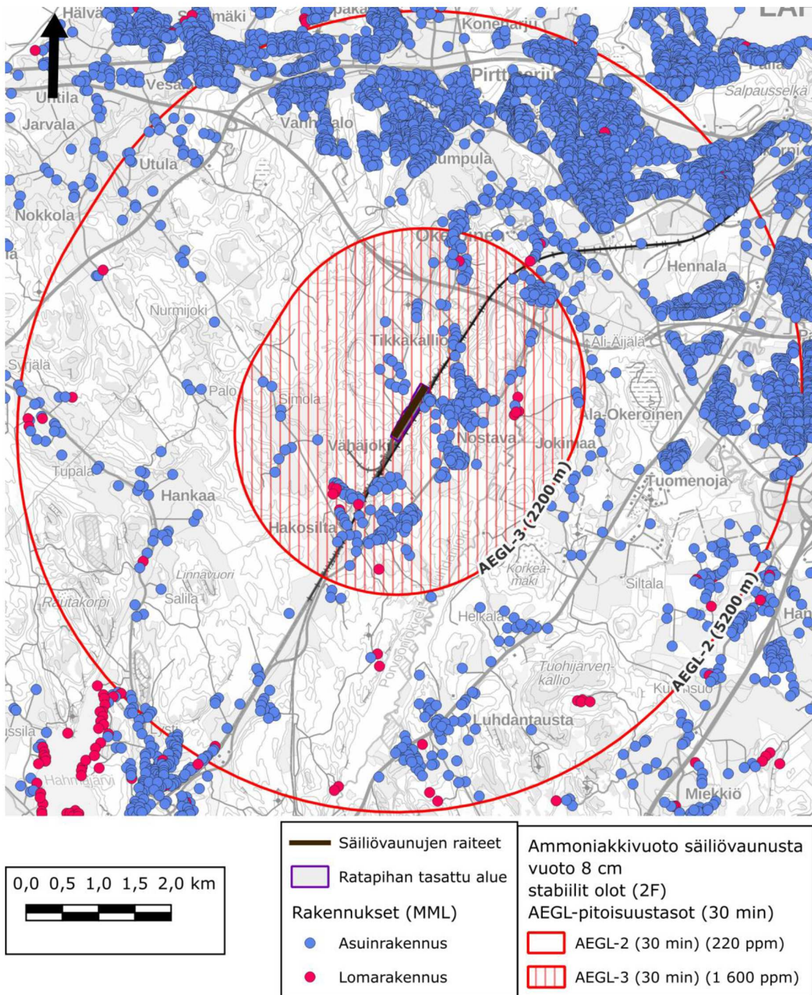
Kuva 39. Ammoniakkivuodon aiheuttamat AEGL-tasojen etäisyydet, kun vedetöntä ammoniakkia vuotaa säiliövaunun pohjalta. Vuodon koko 8 cm, ammoniakkin lämpötila +15 °C. Stabiilit olot (luokka F), tuulen nopeus 2 m/s ja ilman lämpötila +15 °C.
