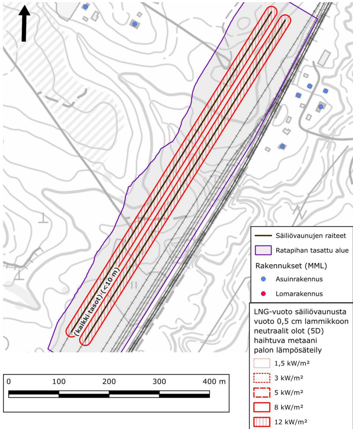
Kuva 22. Lämpösäteilyn tehotasojen vyöhykkeet, kun LNG:n muodostamasta lammikosta haihtuva metaani palaa. Vuodon koko 0,5 cm. Neutraalit olot (luokka D), tuulen nopeus 5 m/s ja ilman lämpötila +15 °C.
