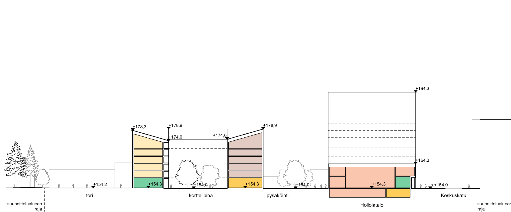
Alueleikkaus A-A 1:750
