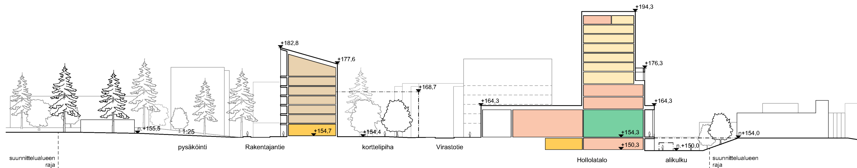
Alueleikkaus B-B 1:750
