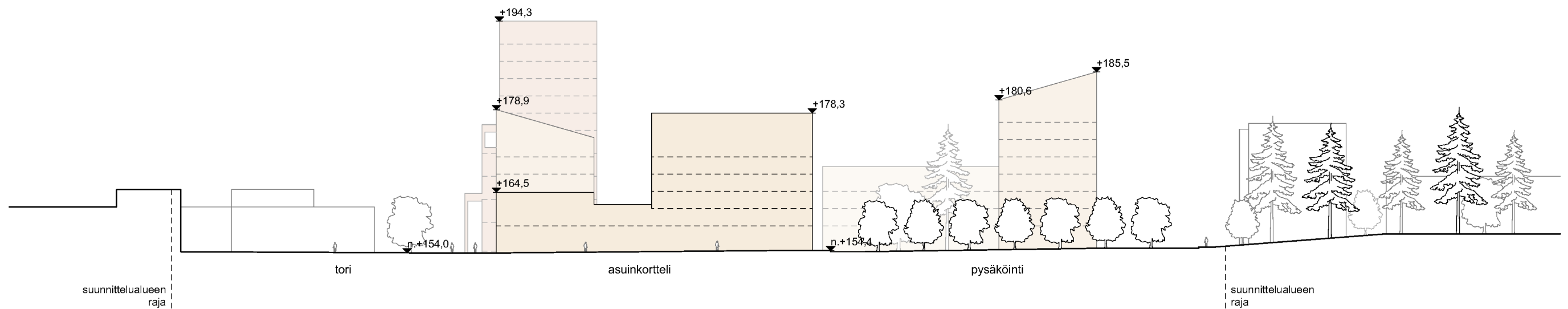
Aluejulkisivu F-F 1:750
