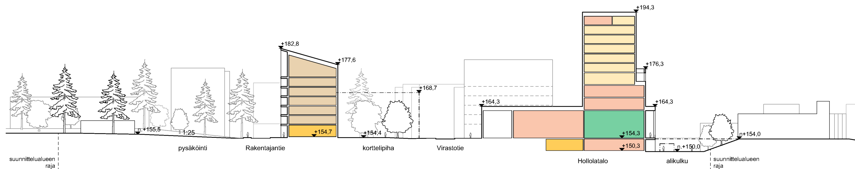
Alueleikkaus B-B 1:750
