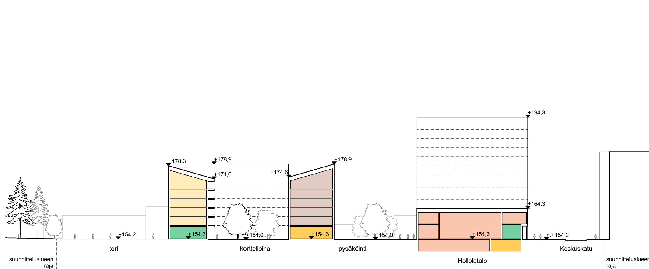
Alueleikkaus A-A 1:750
