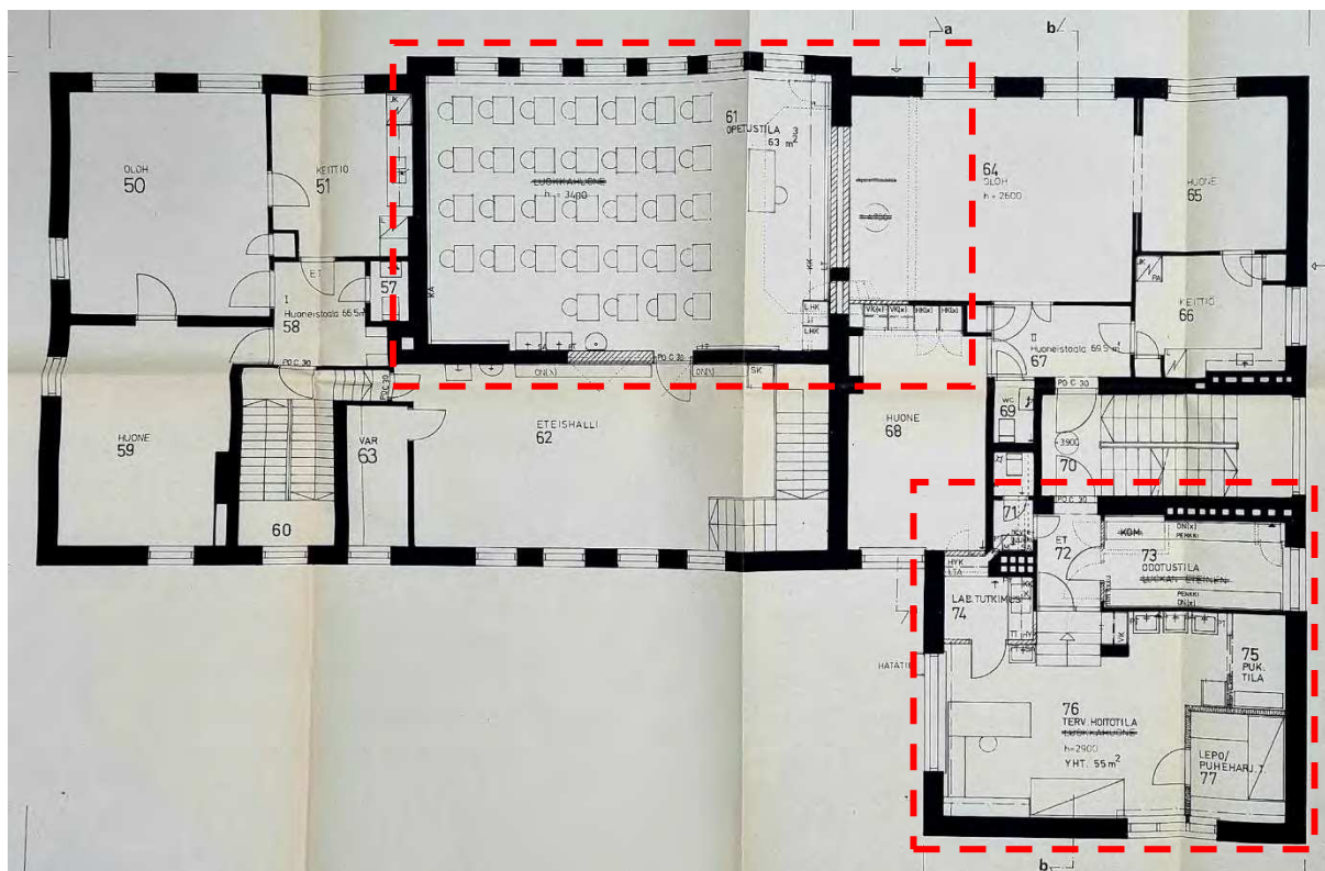
Kuva 34. Toisessa kerroksessa laajennusosan luokkahuone muutettiin terveydenhoitajan tiloiksi, luokkahuoneen näyttämö purettiin ja tila muutettiin osaksi asuinhuoneistoa sekä luokkahuoneen oviaukon paikkaa muutettiin pohjoisemmas. Toisen kerroksen muutospiirustus 2.2.1979, jossa muutosalueet on rajattu punaisella katkoviivalla. (Hollolan rakennusvalvonta)
