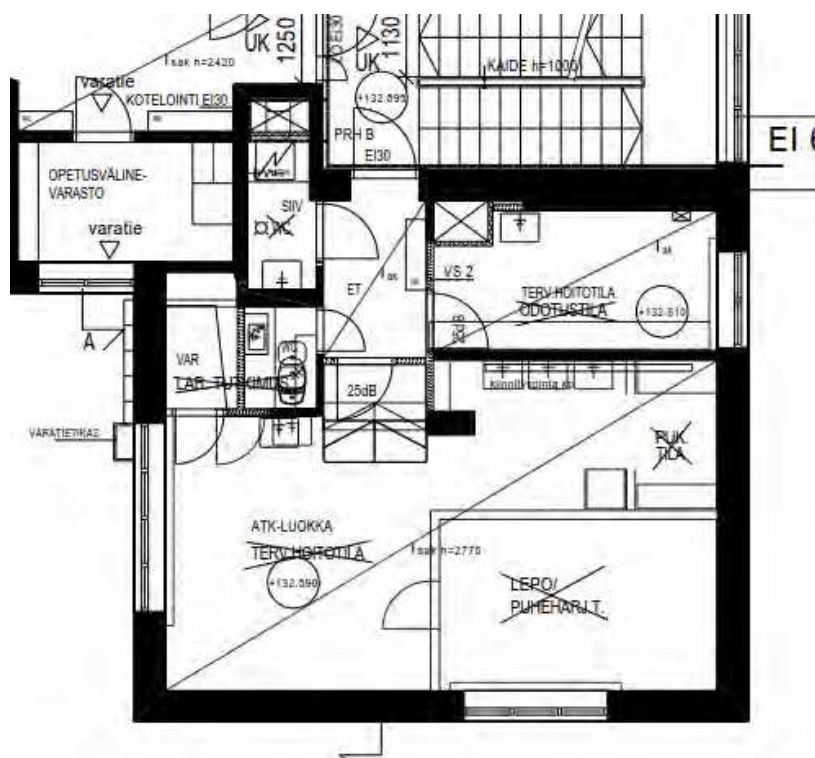
Kuva 42. Pohjoisosan terveydenhoitajan tilat muutettiin luokahuoneeksi ja terveydenhoitajan odotustila säilyi terveydenhoitajan käytössä. Ote muutospirustuksesta 28.11.2001. (Hollolan rakennusvalvonta)
