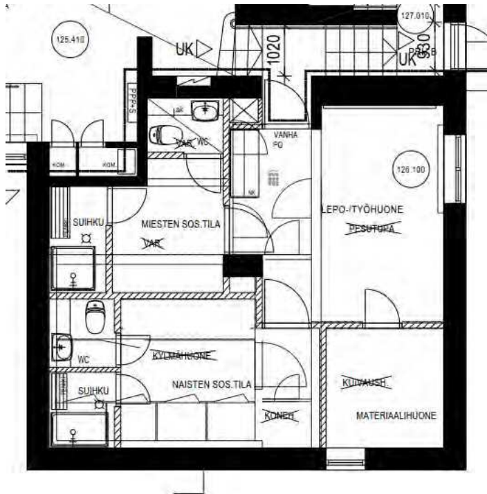
Kuva 44. Pohjoisosan pesutupa, kuivaushuone, kylmähuone ja varastotilat muutettiin lepo- ja työhuoneeksi, materiaalihuoneeksi sekä koulun henkilökunnan sosiaali tiloiksi. Ote muutospirustuksesta 28.11.2001. (Hollolan rakennusvalvonta)
