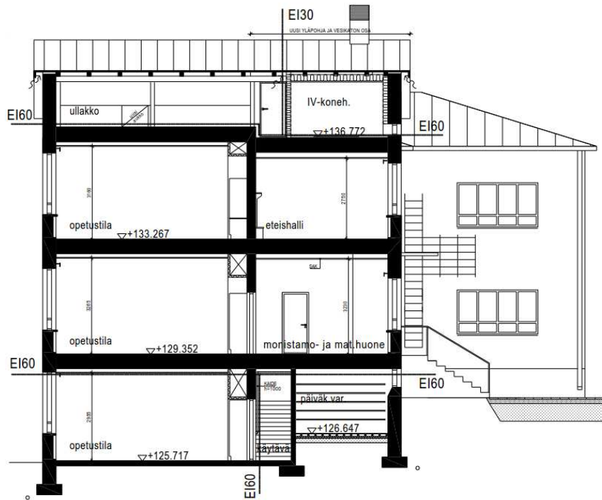
Leikkaus C-C
