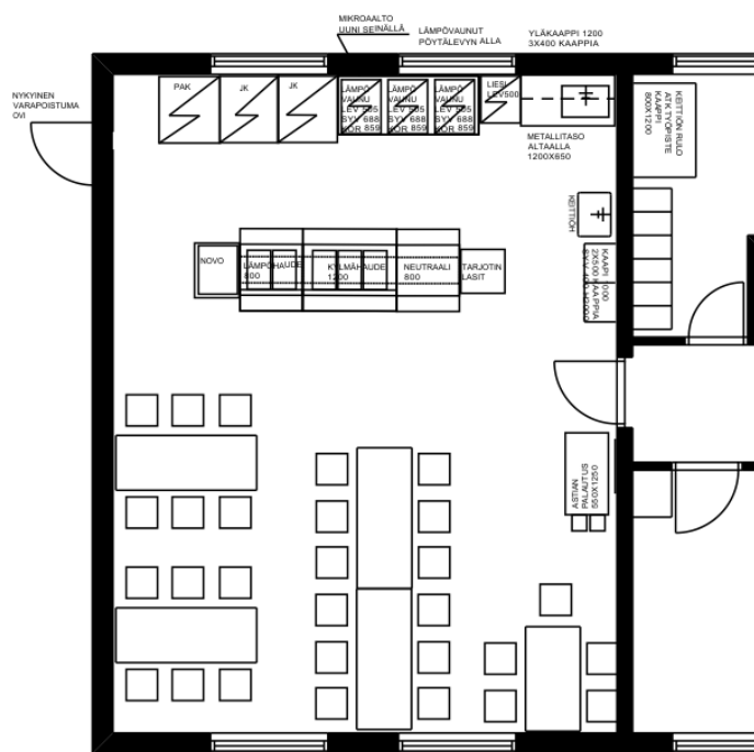
Kuva 51. Puukoulun eteläosaan toteutettiin yhdistetty keittiö ja ruokala. Ote muutospiirustuksesta 8.8.2017. (Hollolan rakennusvalvonta)
