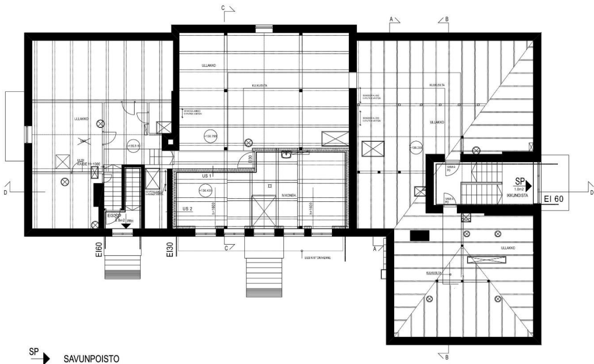
Kuva 45. Ullakkotilaan rakennettiin uusi IV-konehuone. Ote muutospirustuksesta 28.11.2001. (Hollolan rakennusvalvonta)
