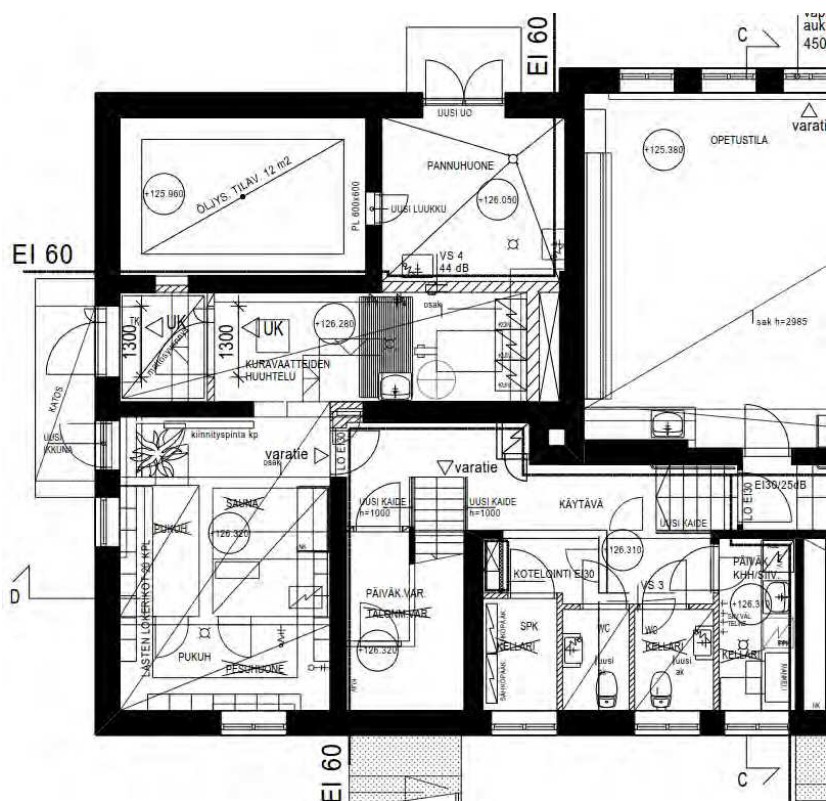
Kuva 43. Kellarikerroksessa eteläosan sauna-, pesuhuone- ja pukuhuonetilat purettiin ja muutettiin päiväkodin eteis- ja vaatesäilytystilaksi. Sisäänkäynnin yhteyteen rakennettiin kuravaatteiden huuhtelu. Keskikäytävän varrella sijainneet tekniset- ja wc-tilat uusittiin. Ote muutospirustuksesta 28.11.2001. (Hollolan rakennusvalvonta)
