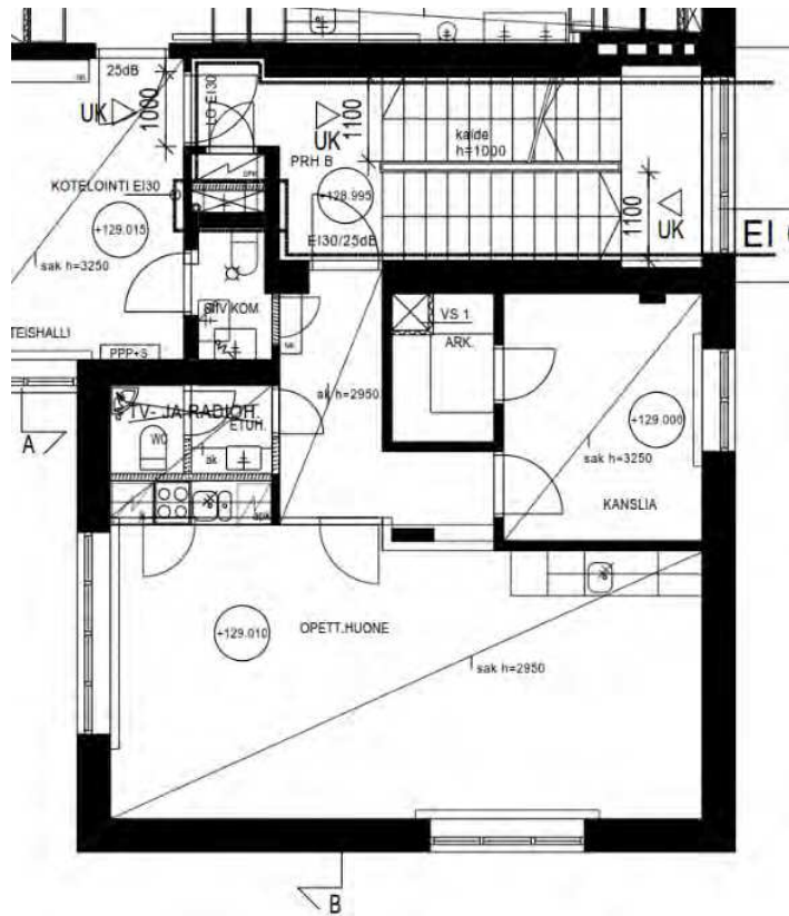
Kuva 40. Ensimmäisen kerroksen pohjoisosassa opettajienhuoneen yhteydessä olleen tv- ja radiohuoneen tilalle rakennettiin wc-tilat. Ote muutospirustuksesta 28.11.2001. (Hollolan rakennusvalvonta)
