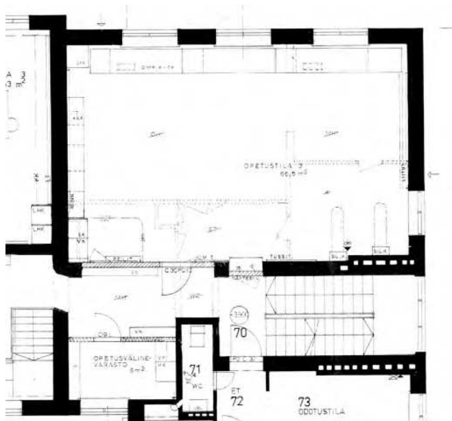
Kuva 37. Laajennusosan toisen kerroksen asunto muutettiin käsityöluokaksi. Ote muutospiirustuksesta 14.12.1987. (Hollolan rakennusvalvonta)
