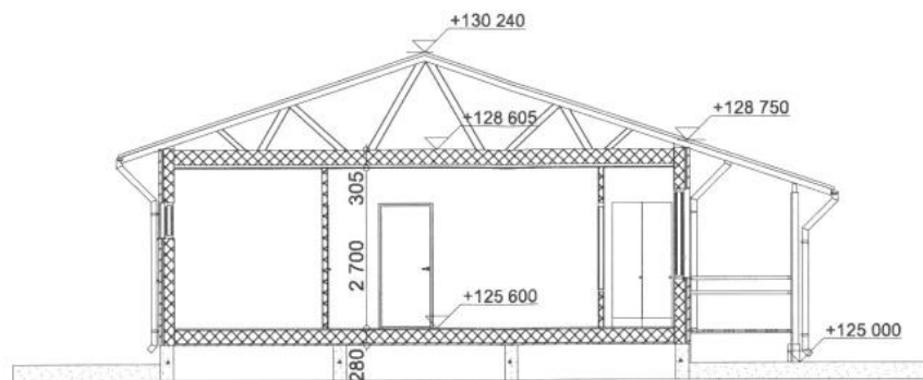
LEIKKAUS A-A
