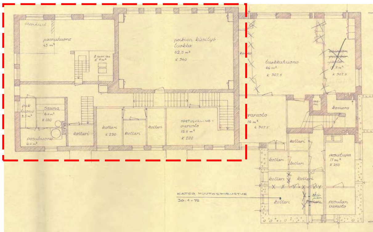
Kuva 15. Pohjapiirustuksesta poiketen eteläsvulle kellarikerrokseen toteutettiin yhden sisäänkäynnin ja kolmen ikkunan sijaan kaksi sisäänkäyntiä ja kaksi ikkunaa. Kellarikerroksen pohjapiirustus vuodelta 1948. Koulun alkuperäinen rakennusosa näkyy kuvassa punaisella katkoviivalla rajattuna. (Hollolan rakennusvalvonta)
