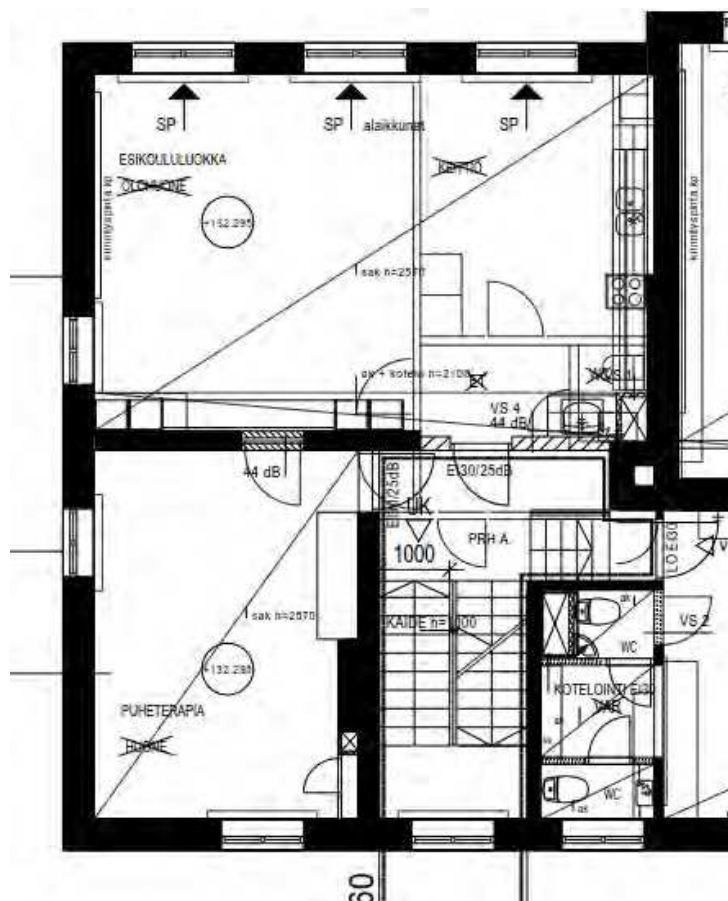
Kuva 41. Toisen kerroksen eteläosan entinen asuinhuoneisto muutettiin esikoululuokaksi sekä puheterapiatilaksi. Ote muutospirustuksesta 28.11.2001. (Hollolan rakennusvalvonta)
