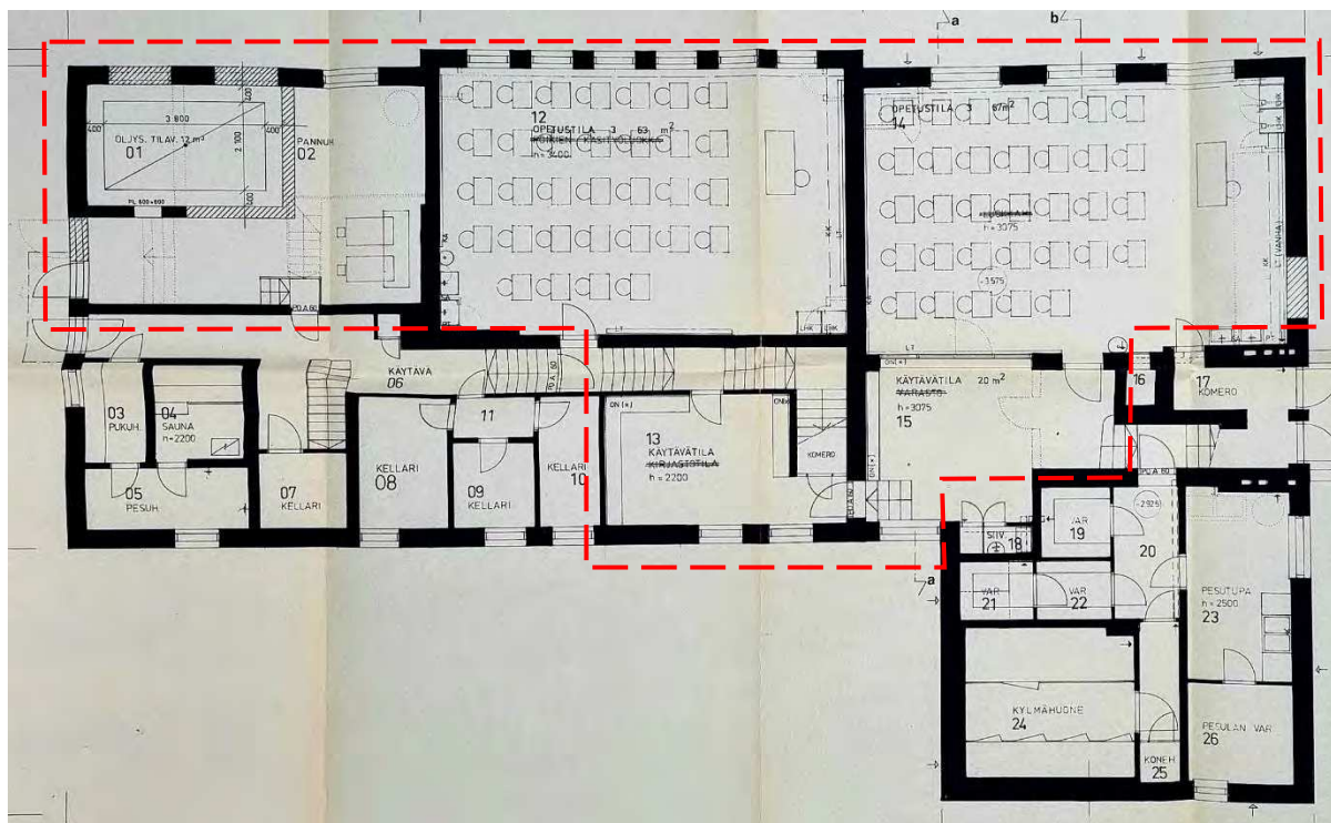
Kuva 35. Kellarikerroksessa olleeseen pannuhuoneeseen toteutettiin tila öljysäiliölle. Kellarikerroksen muutospiirustus 2.2.1979, jossa muutosalueet on rajattu punaisella katkoviivalla. (Hollolan rakennusvalvonta)
