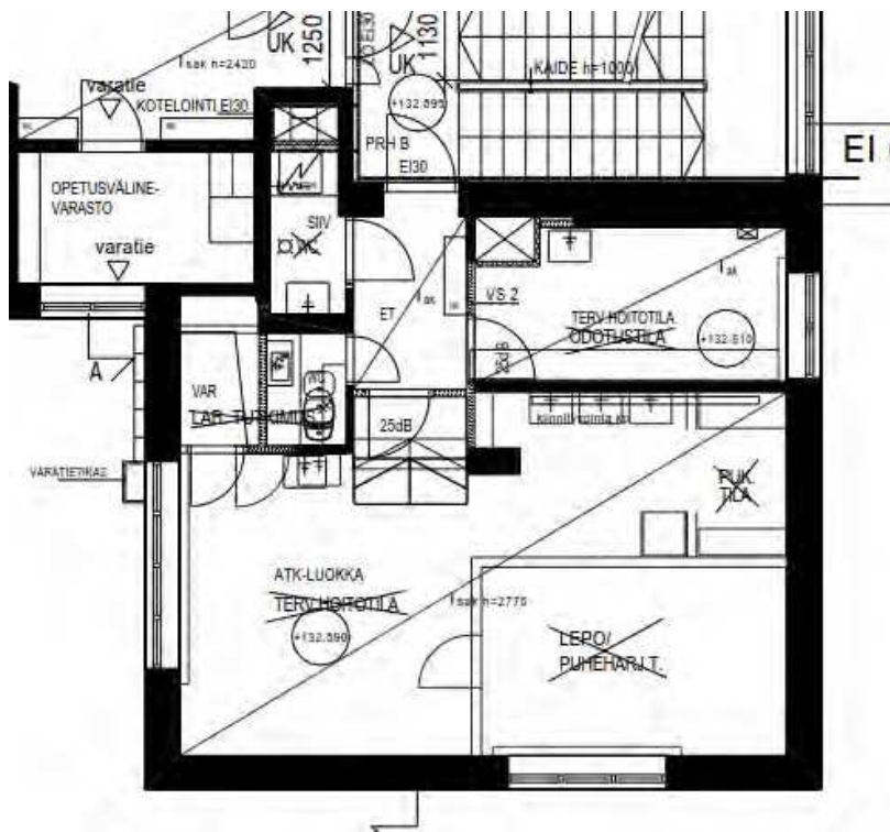
Kuva 42. Pohjoisosan terveydenhoitajan tilat muutettiin luokkahuoneeksi ja terveydenhoitajan odotustila säilyi terveydenhoitajan käytössä. Ote muutospirustuksesta 28.11.2001. (Hollolan rakennusvalvonta)
