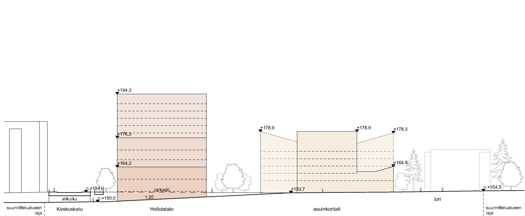
Aluejulkisivu C-C 1:750
