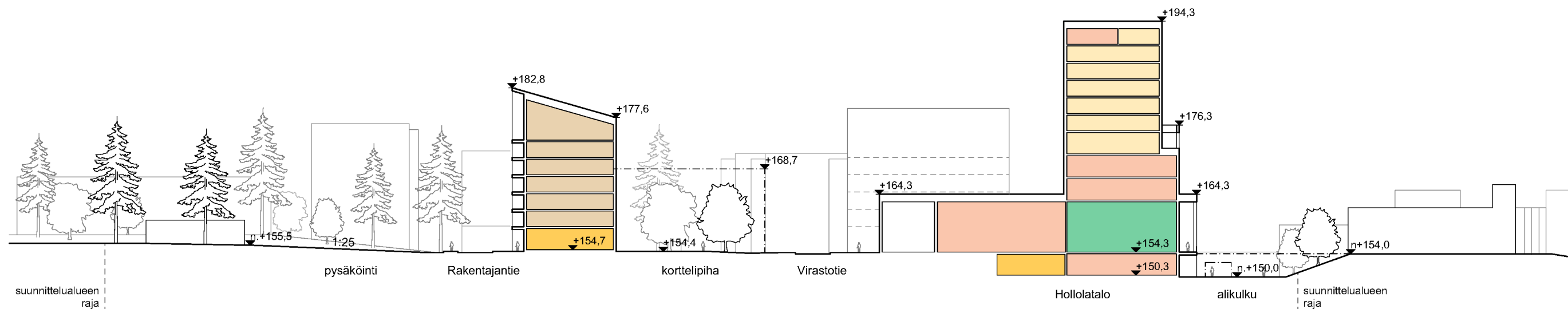
Alueleikkaus B-B 1:750
