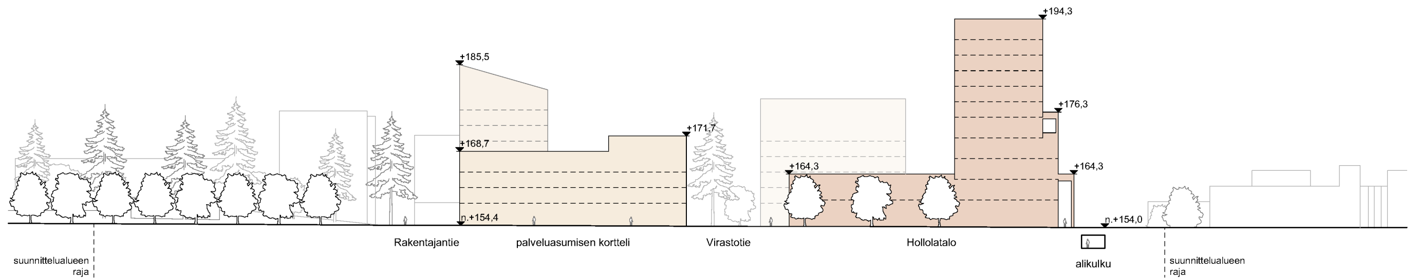
Aluejulkisivu D-D 1:750
