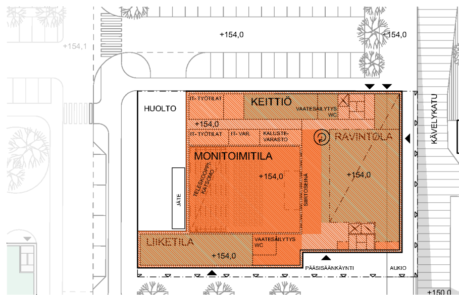
1. kerros 1:750
